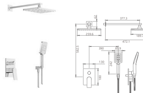
TWL1156A-01 /TWL1156B-01 Two function shower /Finish: CH /MB
