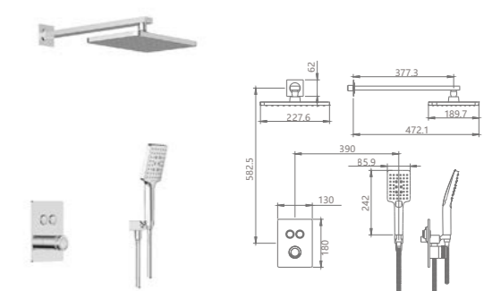
TWL1157A-01 /TWL1157B-01 Two function shower /Finish: CH /MB
